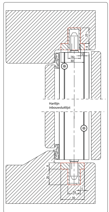
Binnendraaiend RC3
