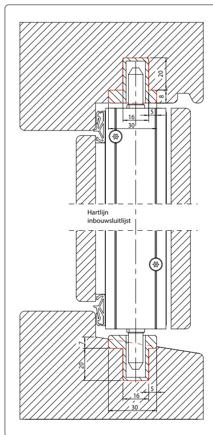
Buitendraaiend RC3
